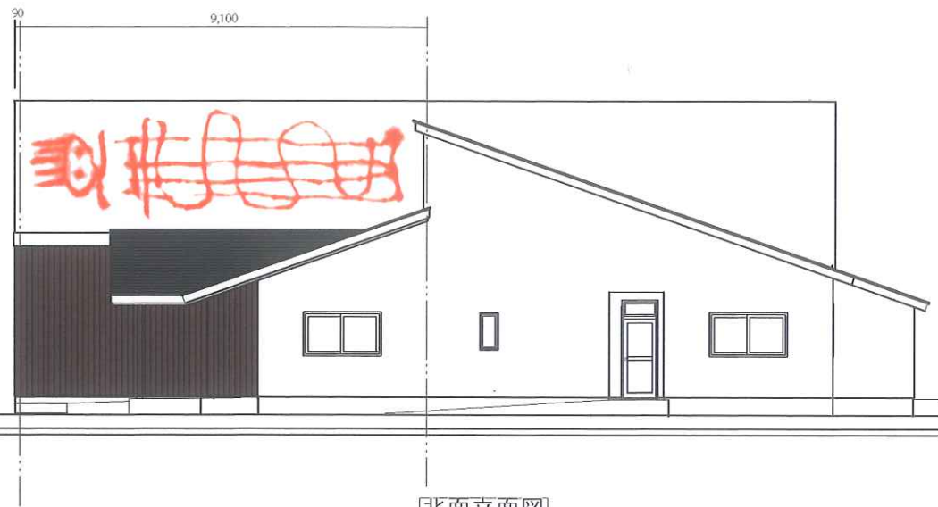
北面立面図
