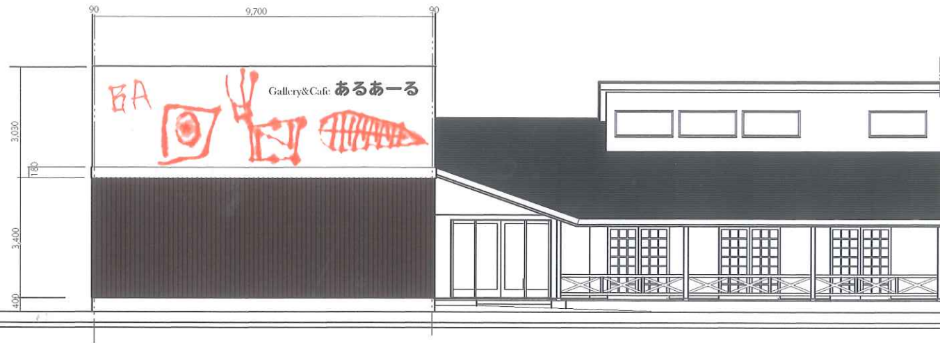
東面立面図
