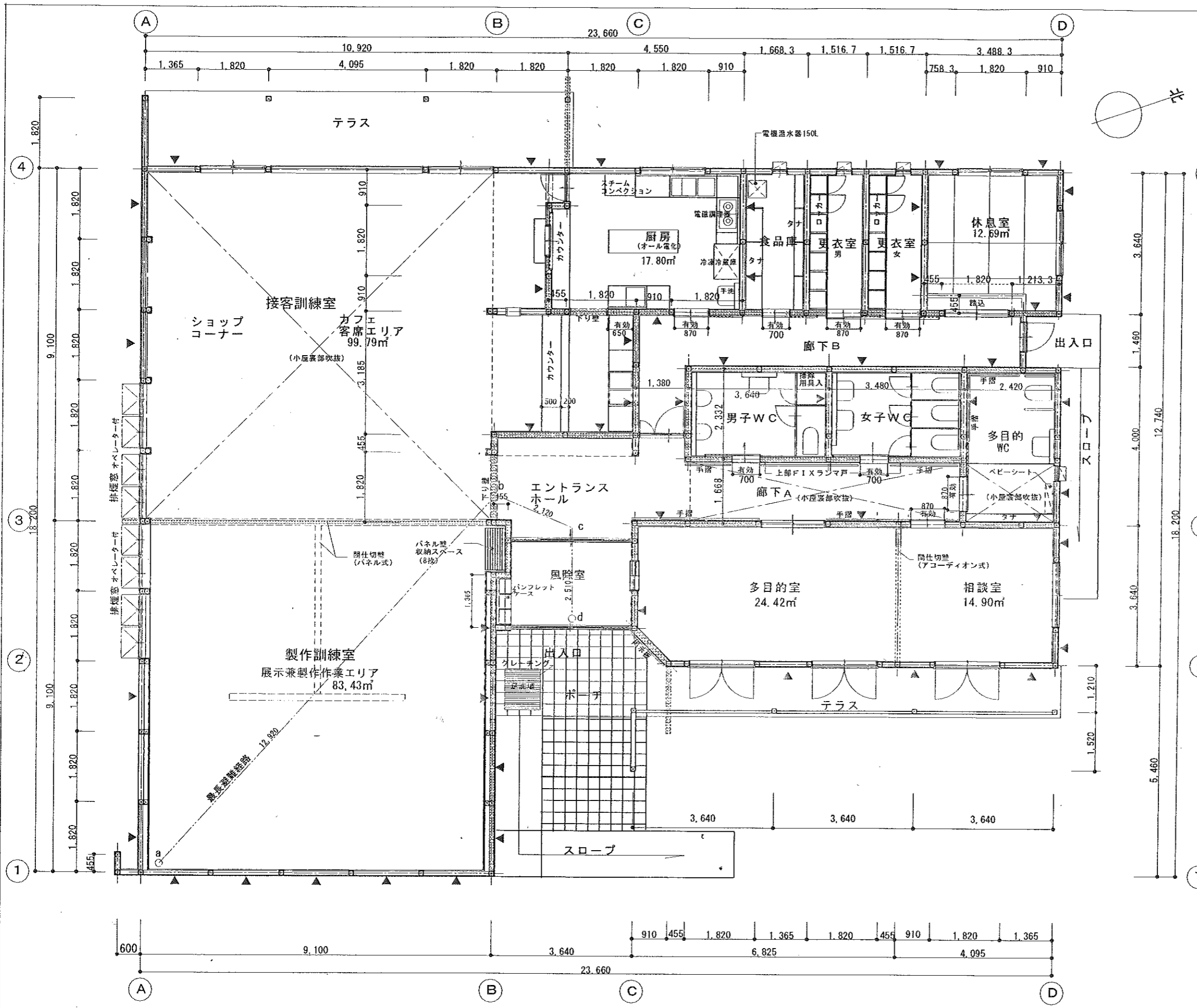
1階平面図 1:100
